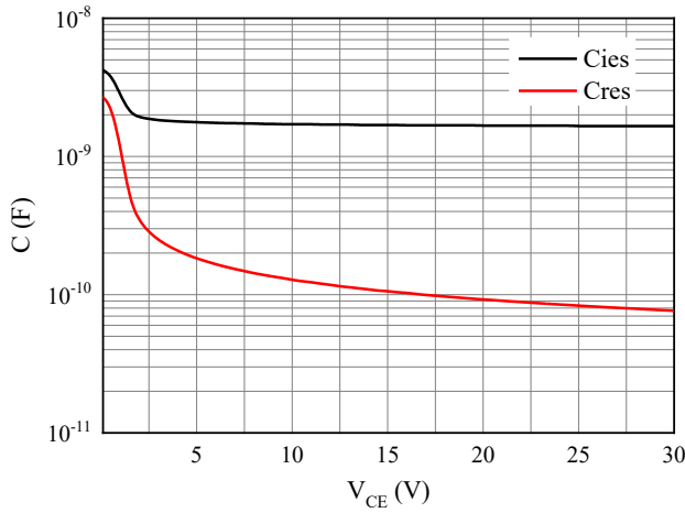
图 9. 电容特性
